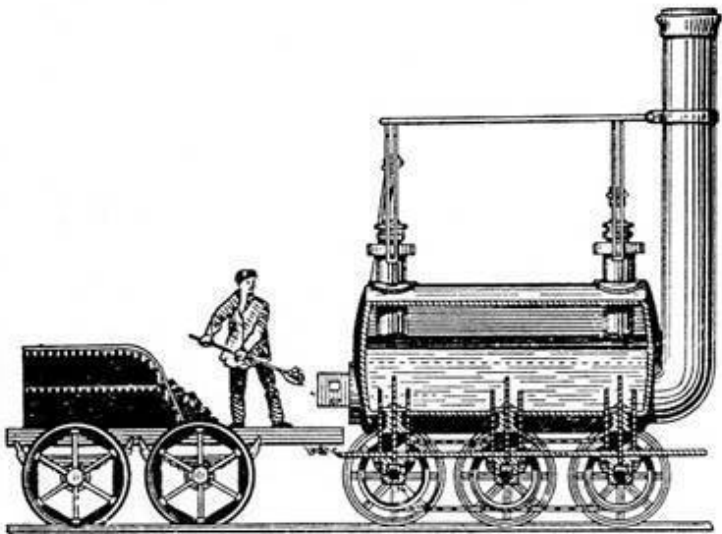
Третий паровоз Дж. Стефенсона "Киллингворт". 1816 год
