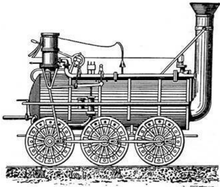
Паровоз Т. Хэкуорта “Августейший Георг”
